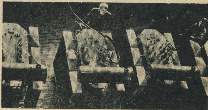
В сборочном цехе завода силовых трансформаторов
